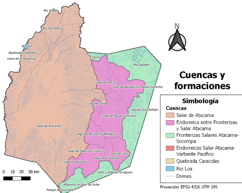
Figura N°4 Hidrografía de la comuna de San Pedro de Atacama.
