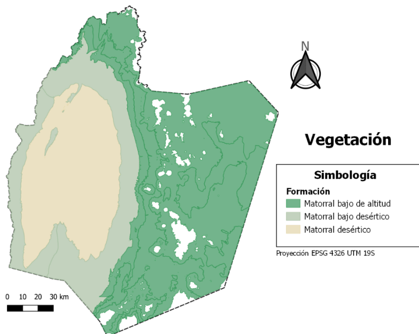
Figura N°7 Vegetación de la comuna de San Pedro de Atacama.
