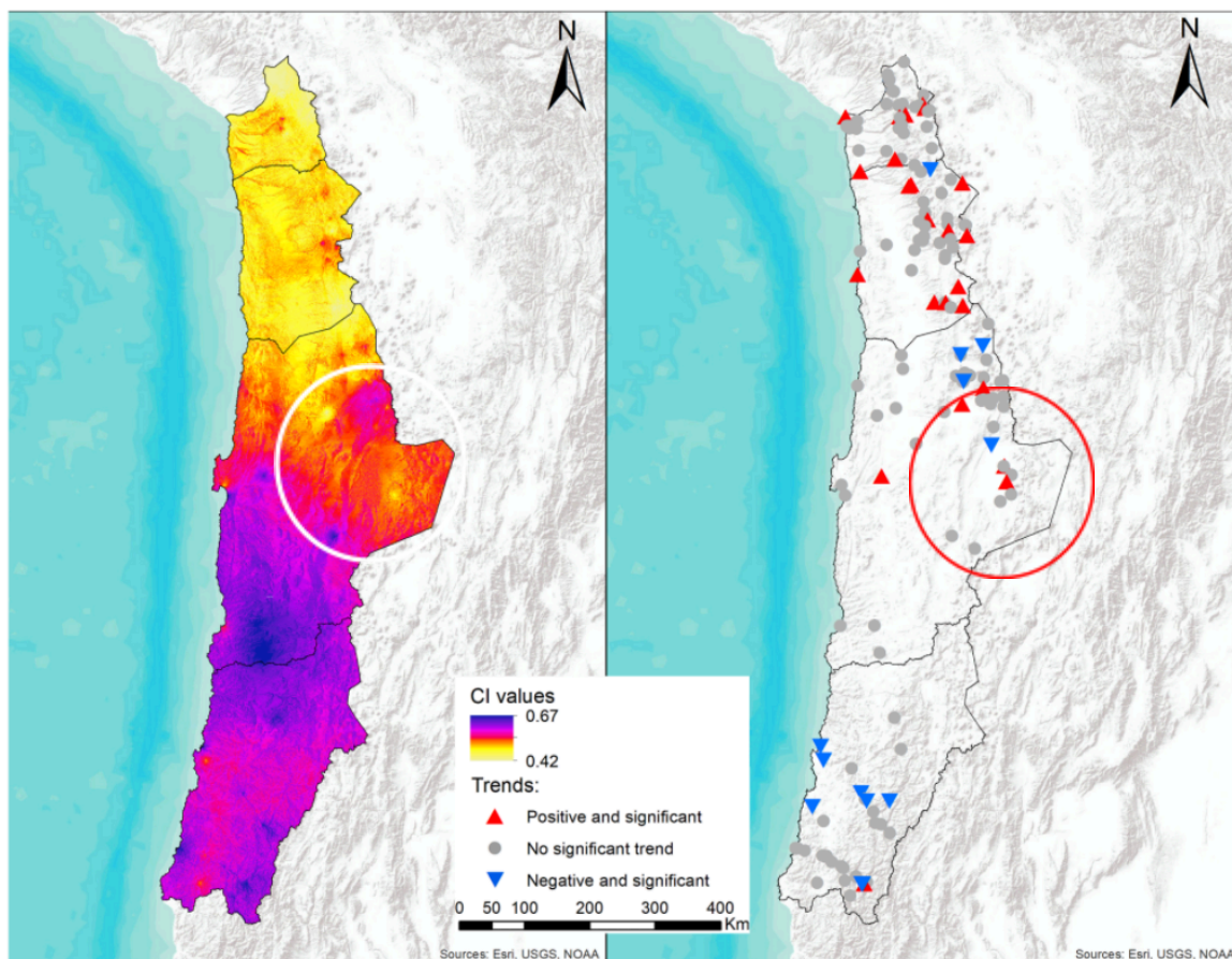
Figura N°21. Índice de Concentración de las precipitaciones.
